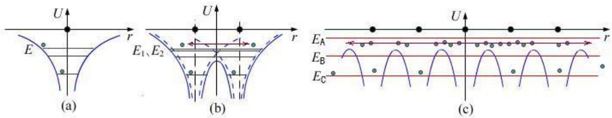
(a) 单个原子能级 E (b) 两个原子 E \rightarrow E_1, E_2 (c) 晶体中的电子共有化，能级分裂成能带
