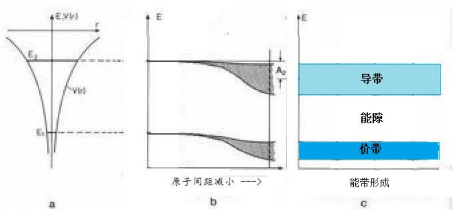
图 2: (a) 单原子能级 (b) 晶体中能级分裂成 N 个 (c) 形成能带
