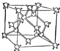
硅晶体的面心立方结构示意图
