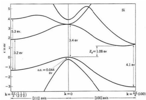
(a) 硅原子的能带图
