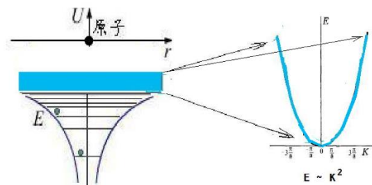
(b) 自由电子的能带
